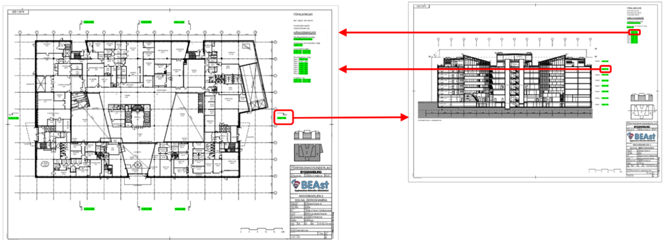
(Figur: Hänvisningar från plan till sektion enligt BEAst (exempel 2))
