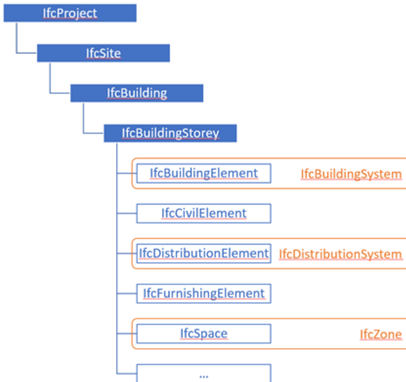
(Figur: IFC entitets i trädstruktur)
