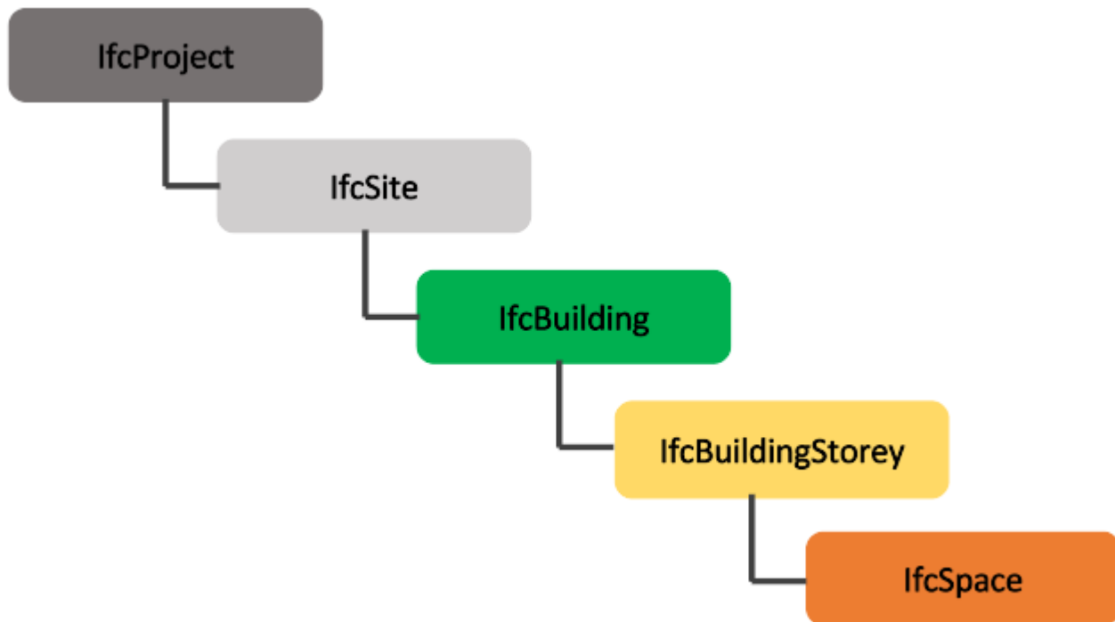
Figur 2: Rumslig hierarki av byggnader i IFC.
